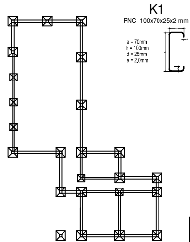
PLANTA DE FUNDACIONES
